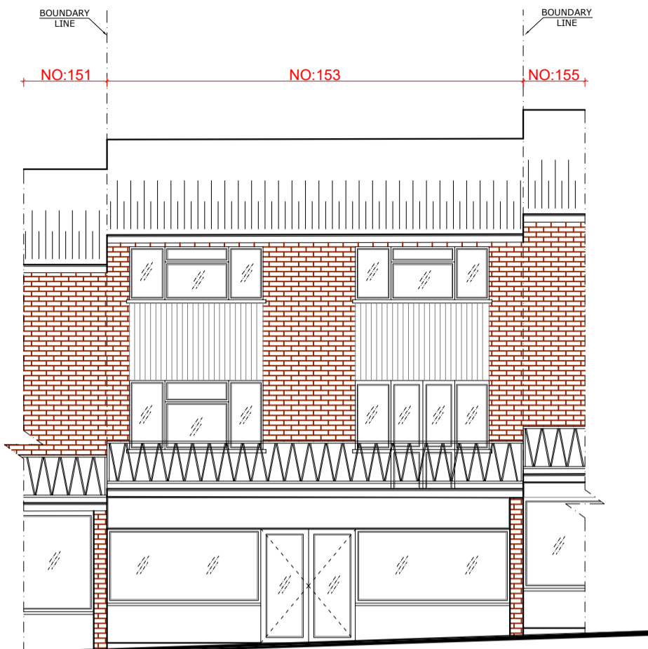
EXISTING FRONT ELEVATION SCALE: 1/100 @A3
