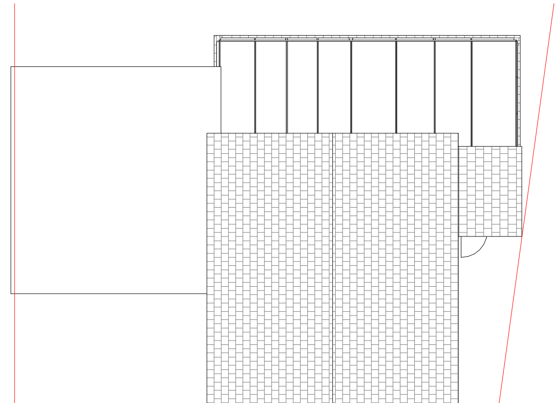
02 - Roof Plan 1 : 100
