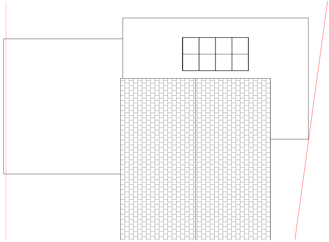
02 - Roof Plan 1 : 100
